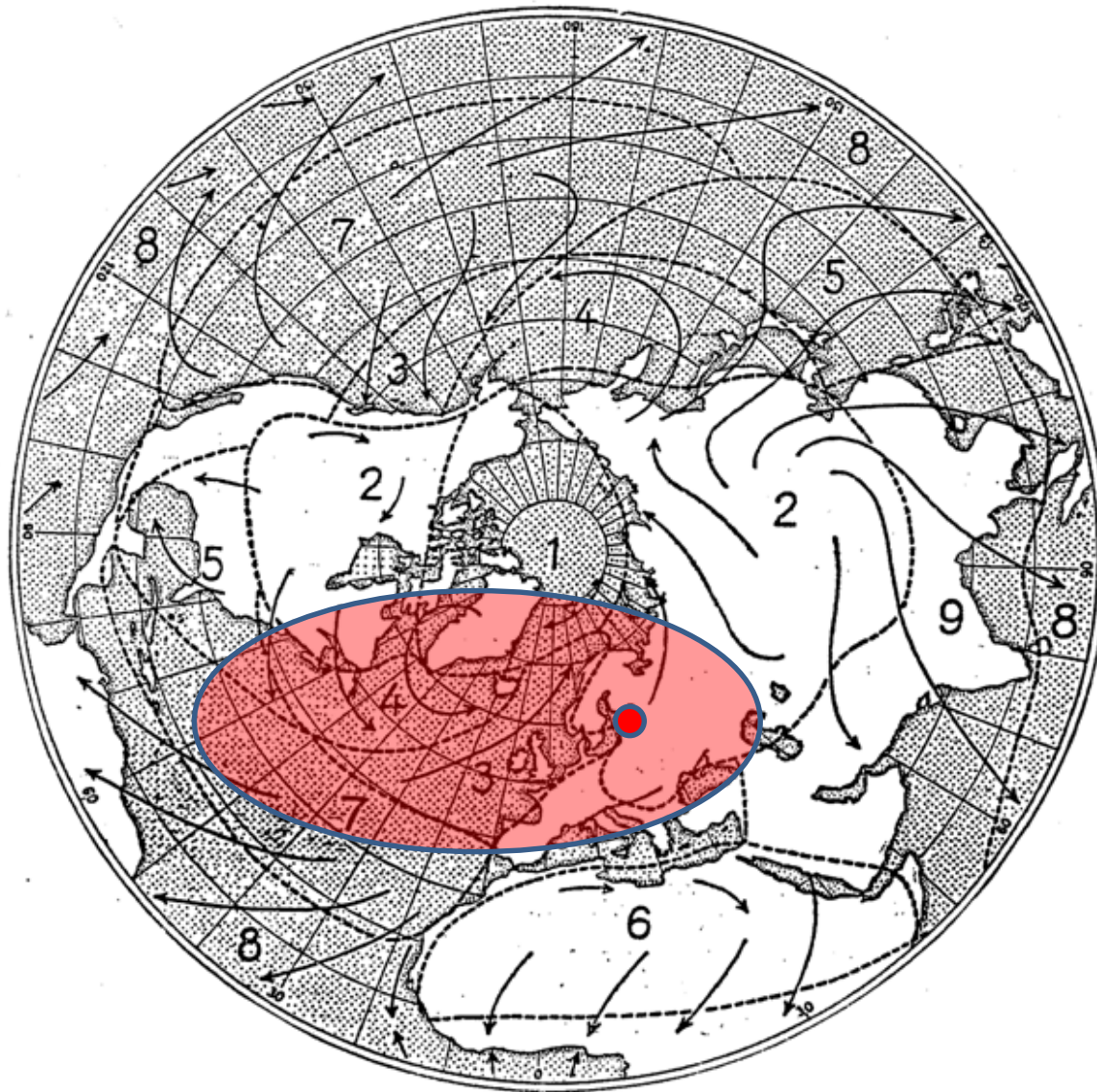
Joonis 1. Õhumasside kolded talvisel ajal põhjapoolkeral.
